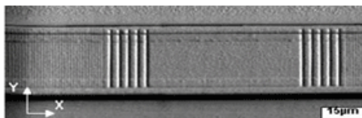
Image d'un sNSOM à basse température (Appl. Phys. Lett. 98, 231112 (2011)).
